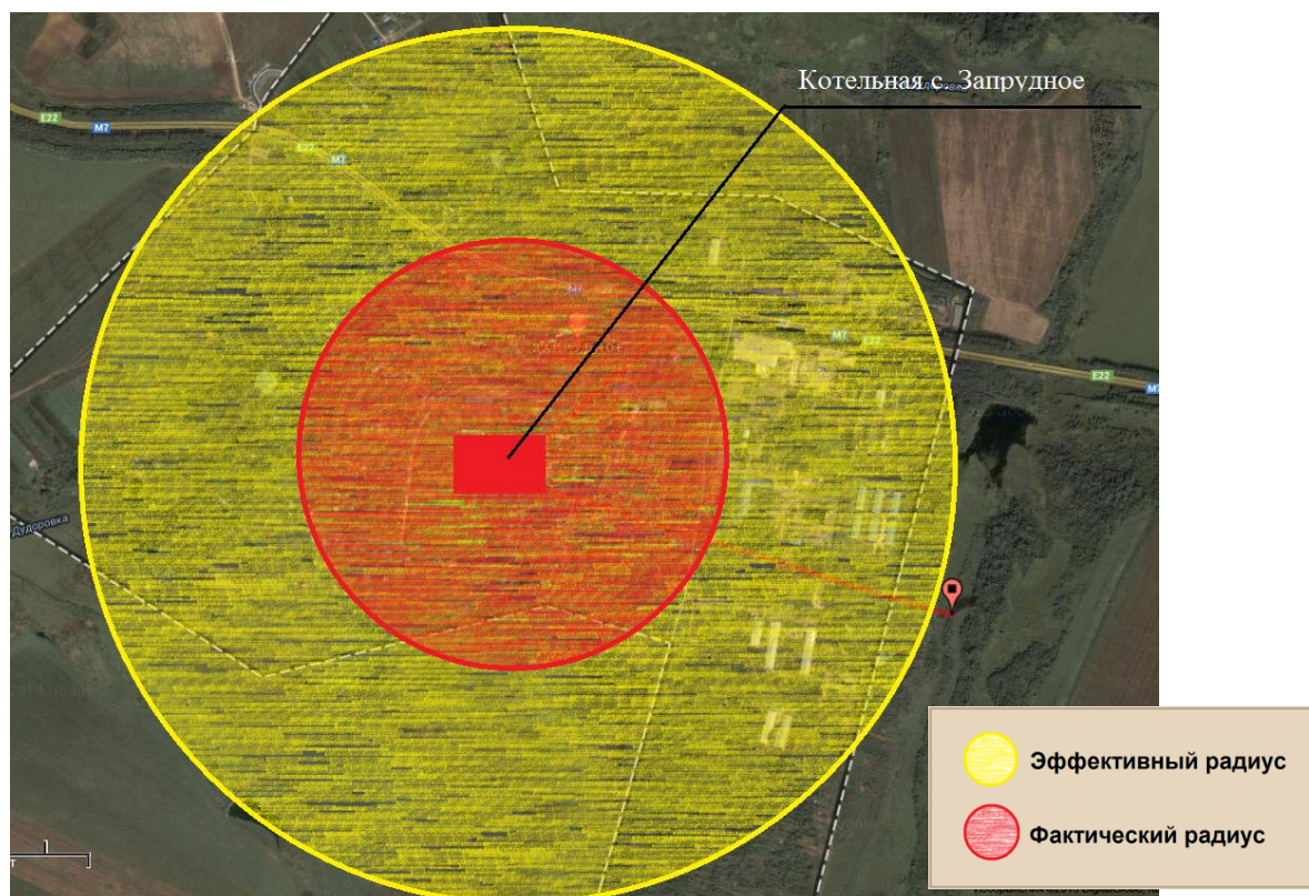
2.1.1 Эффективный радиус теплоснабжения котельной с. Запрудное
