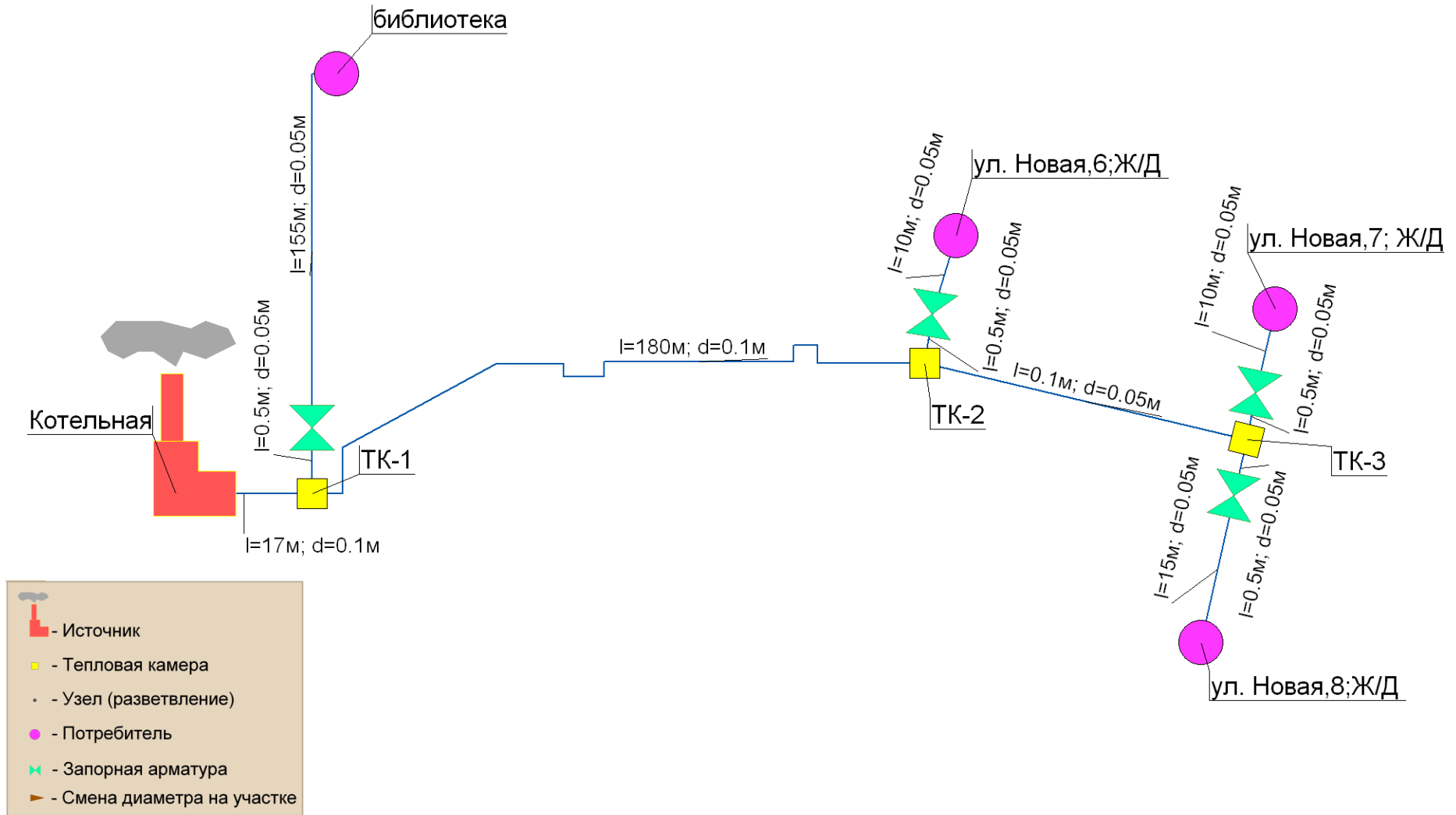
Рис. В4.2. Схема тепловой сети в зоне действия котельной с. Шава
